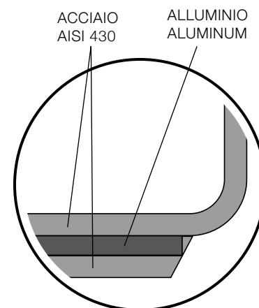
Fondo termodiffusore Thermal diffusion bottom
